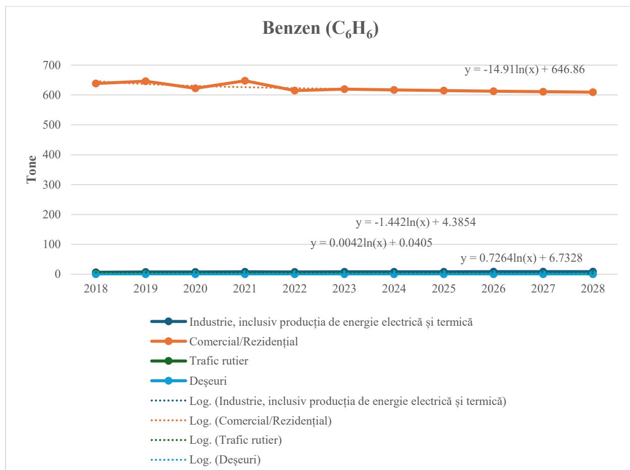
Figura 49- Tendința cantităților de benzen ( C_6H_6 ) la nivelul județului Dâmbovița în perioada de proiecție 2024-2028 – Scenariul de bază (Sursa date: Inventarele locale de emisii ale județului Dâmbovița 2018-2022, APM Dâmbovița)
