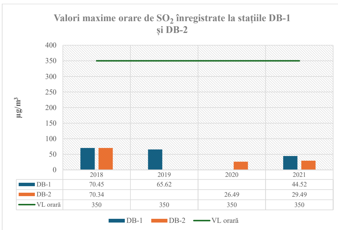
Figura 18- Concentrații maxime orare de \text{SO}_2 în perioada 2018-2021 în județul Dâmbovița (Sursa date: calitateaer.ro )
