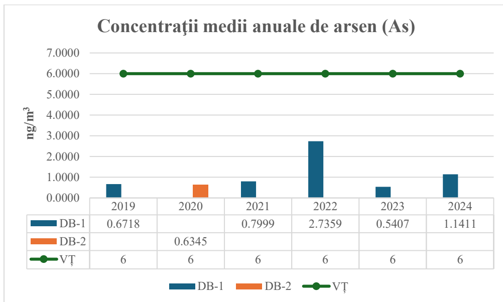
Figura 22 – Concentrații medii anuale de arsen (As) raportate la valoarea țintă pentru conținutul total din fracția PM10, mediată pentru un an calendaristic în perioada 2019-2024 (Sursa: DJM Dâmbovița)
