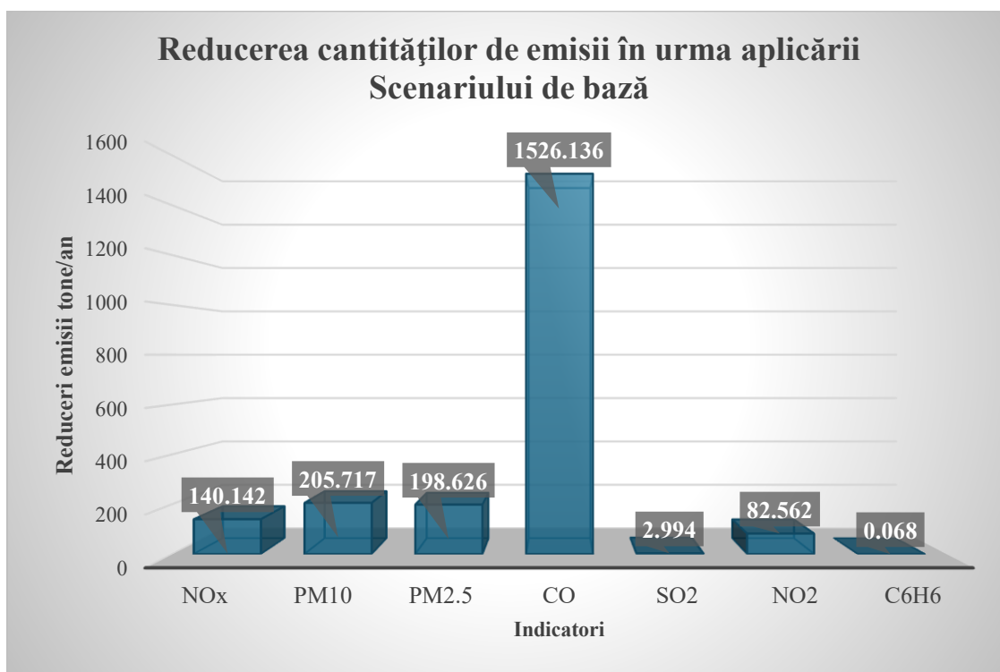
Figura 54- Reducerea cantităților de emisii pentru indicatorii CO, C 6 H 6 , NO 2 , SO 2 , NO x , PM 10 , PM 2.5 în urma aplicării Scenariului de bază
