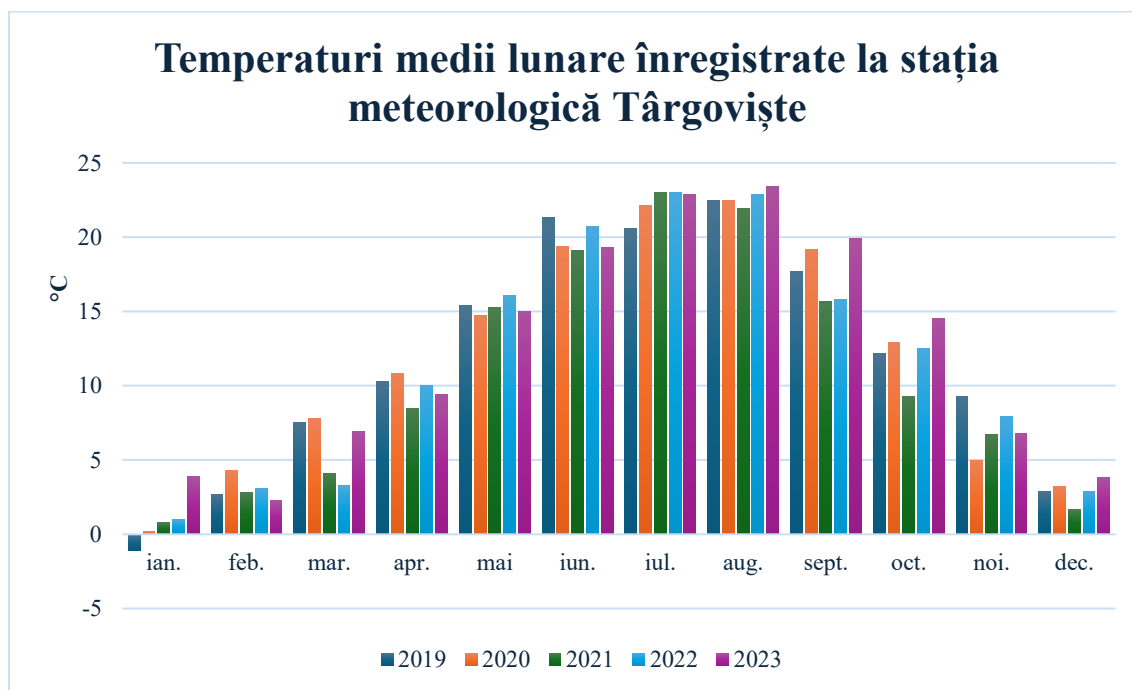
Figura 3- Temperaturi medii lunare înregistrate în perioada 2019 - 2023 la stația meteorologică Târgoviște (Sursă date: Administrația Națională Oceanică și Atmosferică a Statelor Unite ale Americii, prin accesarea bazei de date online - NOAA – https://www.ncdc.noaa.gov/cdo-web/datasets )
