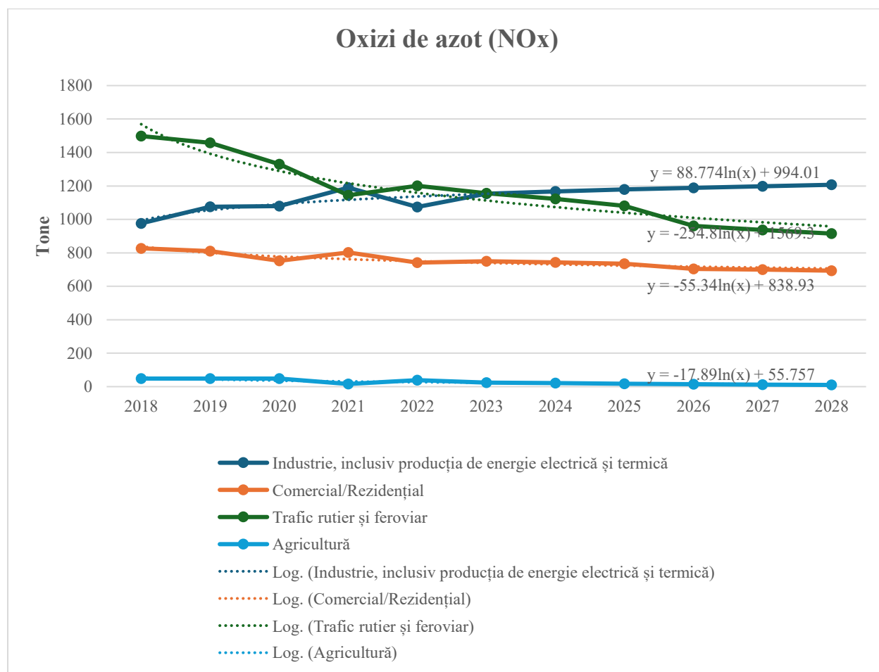
Figura 45- Tendința cantităților de oxizi de azot (NOx) la nivelul județului Dâmbovița în perioada de proiecție 2024-2028 – Scenariul de bază (Sursa date: Inventarele locale de emisii ale județului Dâmbovița 2018-2022, APM Dâmbovița)
