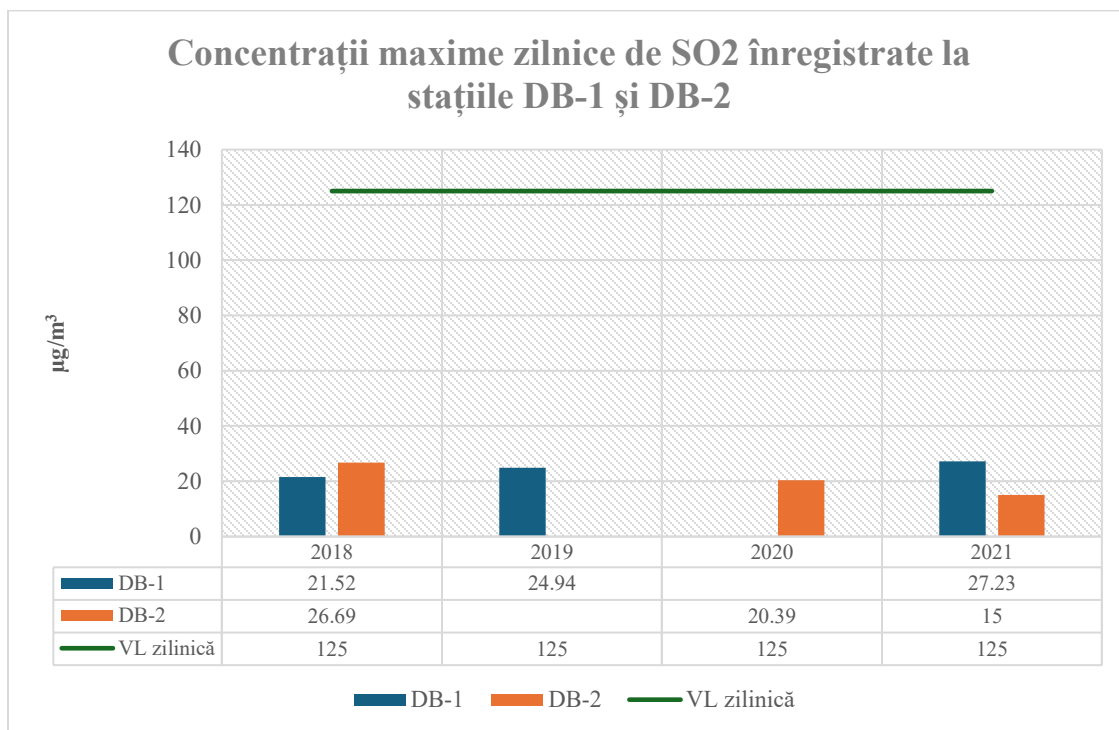
Figura 17- Evoluția concentrațiilor maxime zilnice de SO 2 înregistrate la stațiile DB-1 și DB-2 în perioada 2018-2021 (sursă date: calitateaer.ro)
