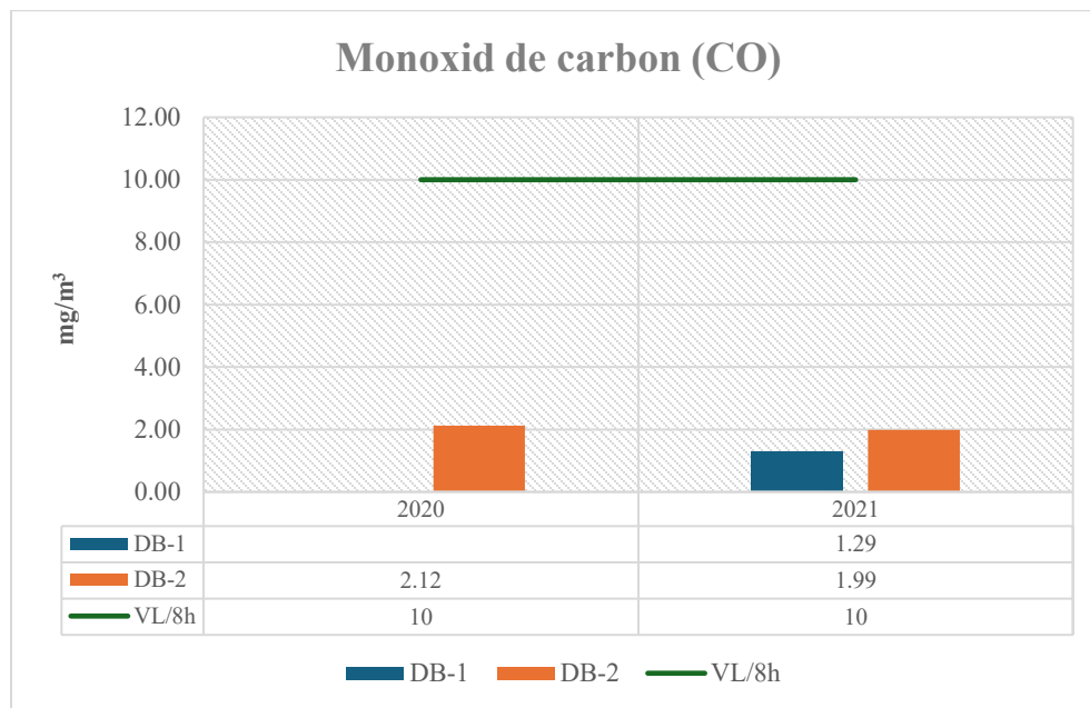
Figura 16- Maxima zilnică a mediei pe 8 ore a indicatorului monoxid de carbon (CO) în perioada 2020-2021 în județul Dâmbovița (Sursă date: calitateaer.ro)
